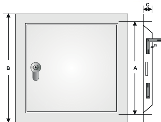
A = objednávaci rozmer B = rozmer A+35 mm C = 25 mm
